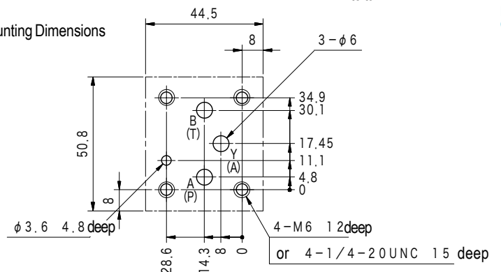
DT1M2
