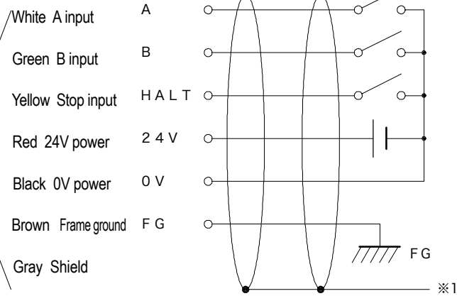
Color Wire Function Nomenclature
